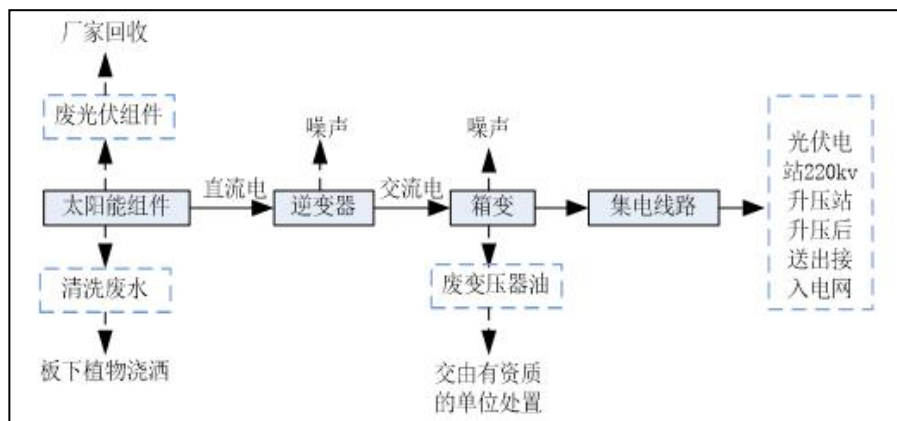
图 4-2 运营期产污环节示意图
