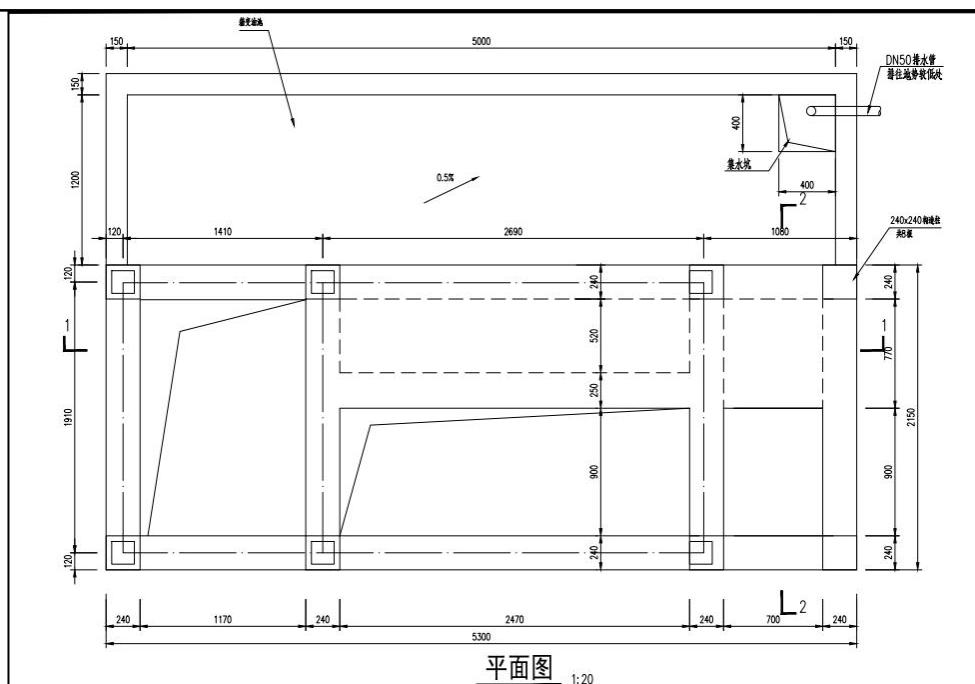
图 2-4 箱式变压器基础体型图
