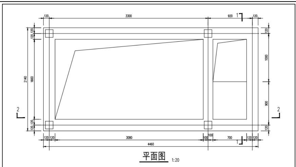
图 2-5 电缆分接箱基础体型图
