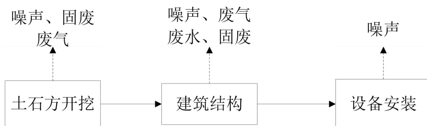
图 2-2 污水处理厂施工期产污节点图
