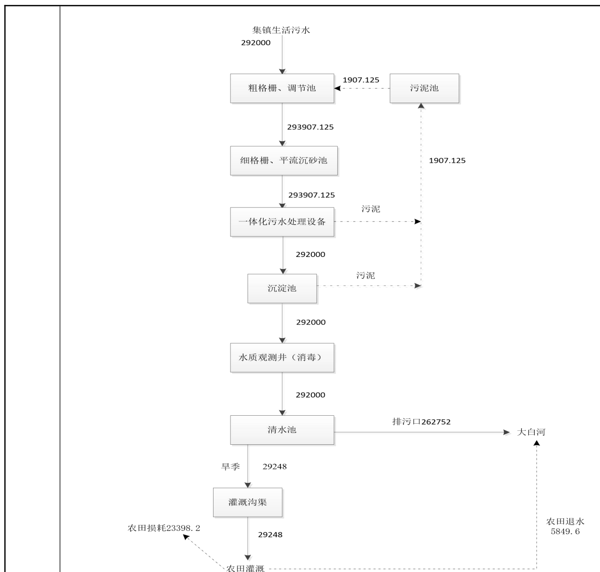
图 2-1 全年水量平衡图 单位：m³/a
