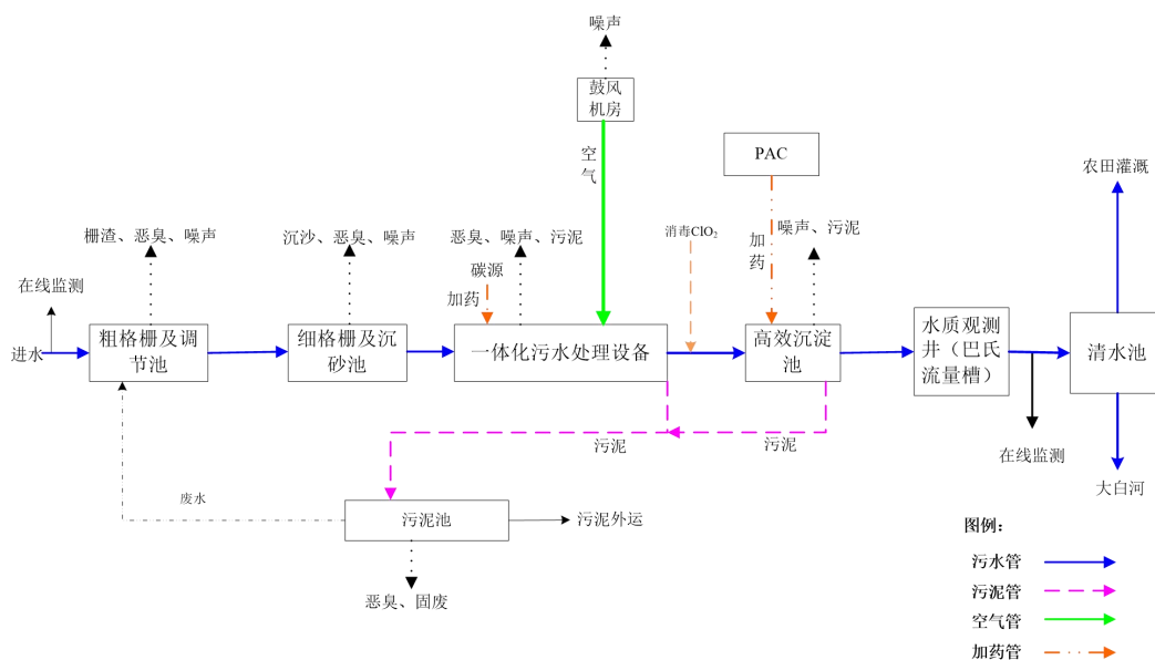
图 2-4 工艺流程及产物节点
