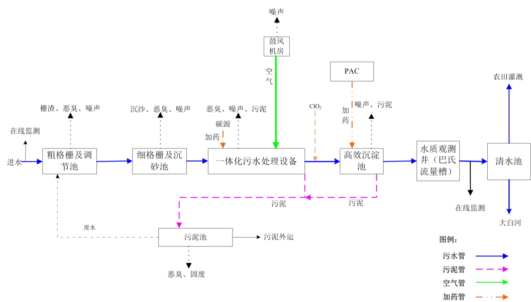
图 2-6 工艺流程及产污节点
