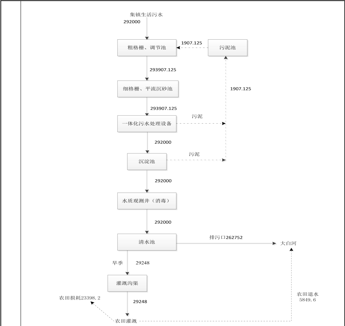
图 2-3 全年水量平衡图 单位：m³/a
