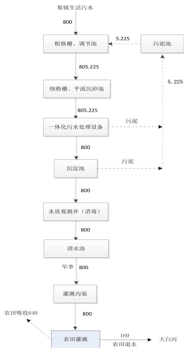
图 2-1 非雨天灌溉时水量平衡图 单位: \text{m}^3/\text{d}
