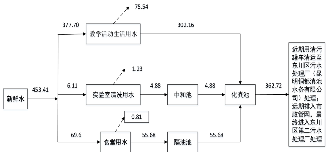
图 2-2 项目运营期雨天水平衡图 (m³/d)
