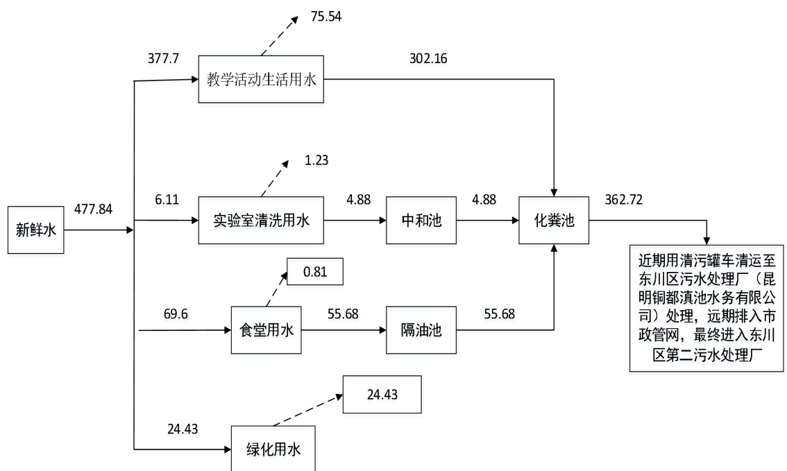
图 2-3 项目运营期非雨天水平衡图 (m³/d)
