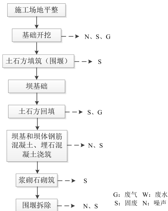
图2.10-1 取水坝/挡水坝施工工艺流程图
