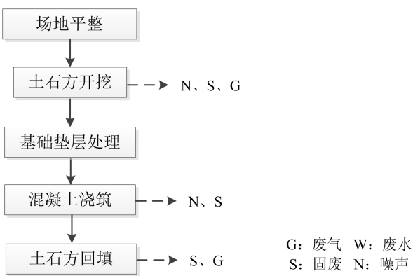
图2.10-4 水池施工工艺流程图
