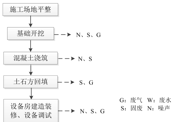
图 2.10-2 设备房施工工艺流程图
