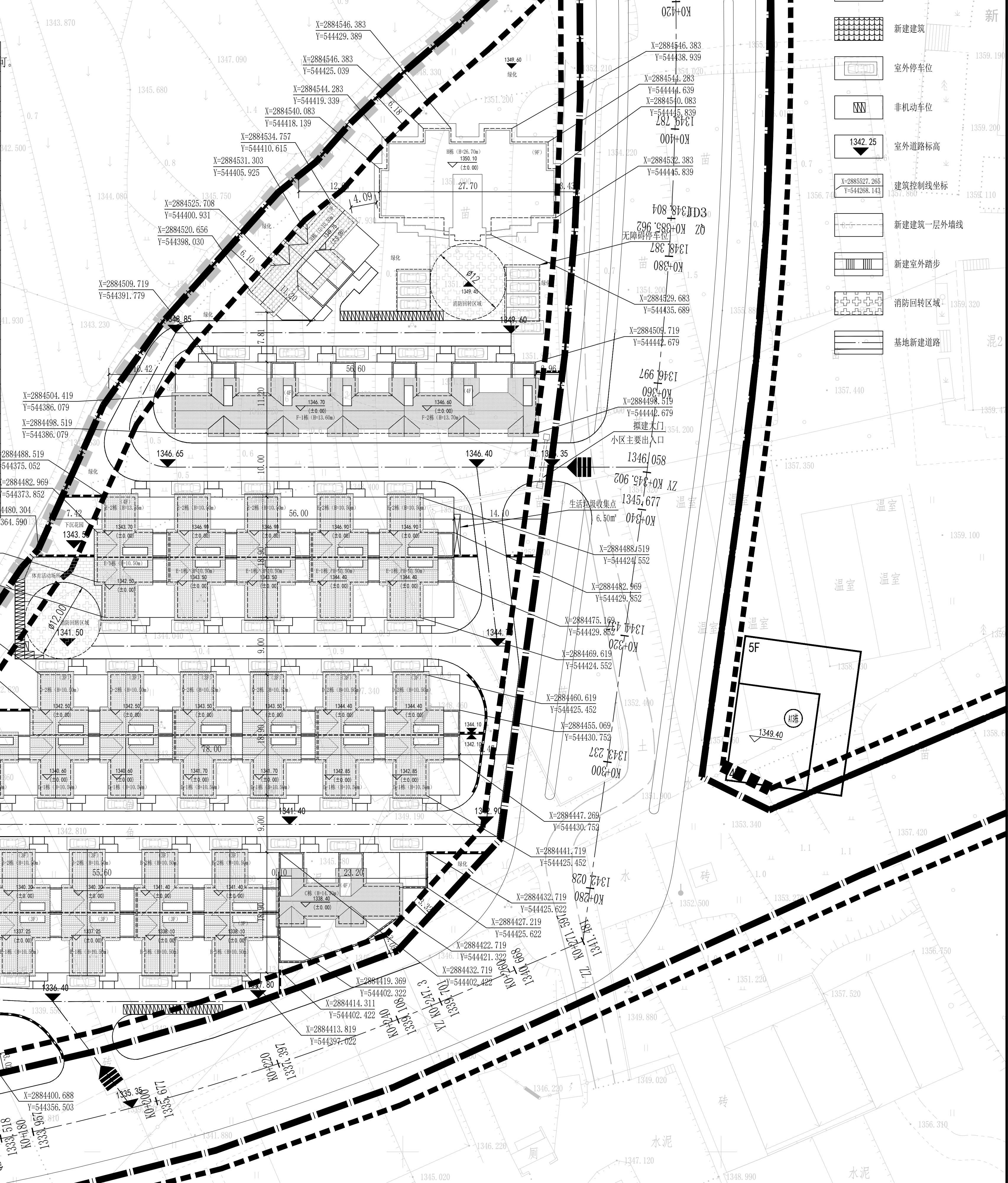
总平面定位布置图 1:500
