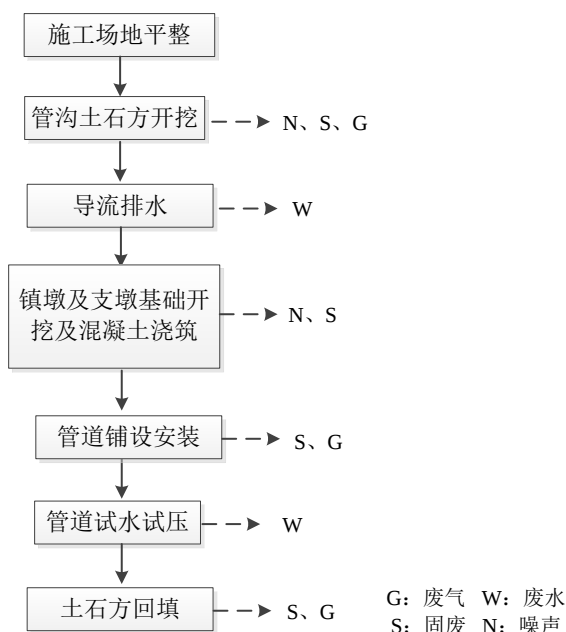
图 2.10-3 管道施工工艺流程图
