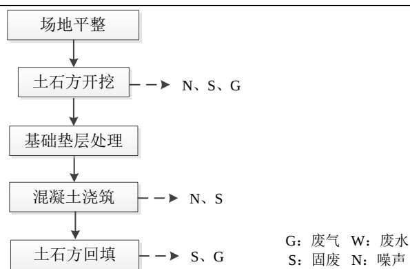
图2.10-4 水池施工工艺流程图
