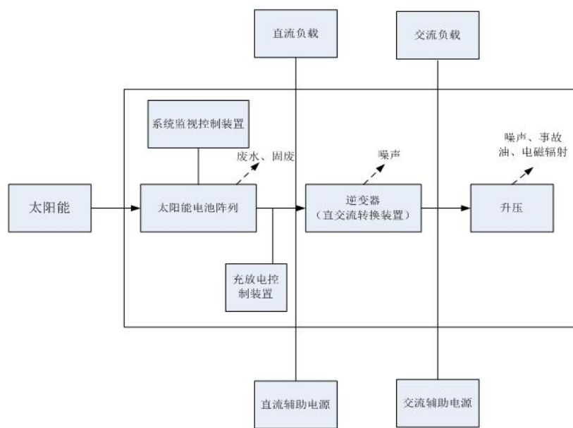
图4-3 运行期太阳能光伏阵列产污环节图
