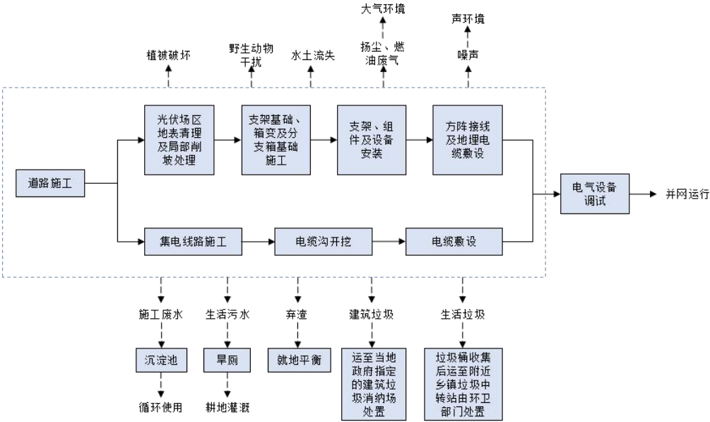
图4-1 光伏发电系统施工工艺流程及产污环节图
