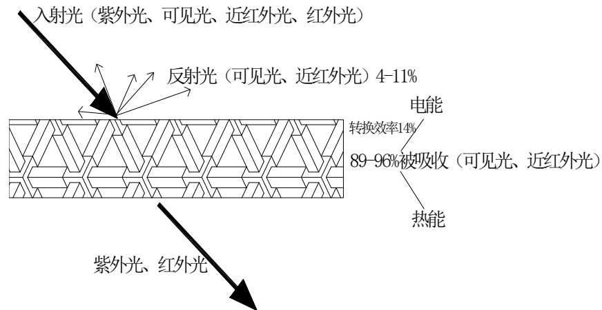
图4-4 太阳能电池反射示意图
