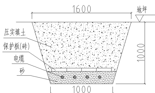
图 2-5 直埋电缆典型横剖面图（单位：mm）
