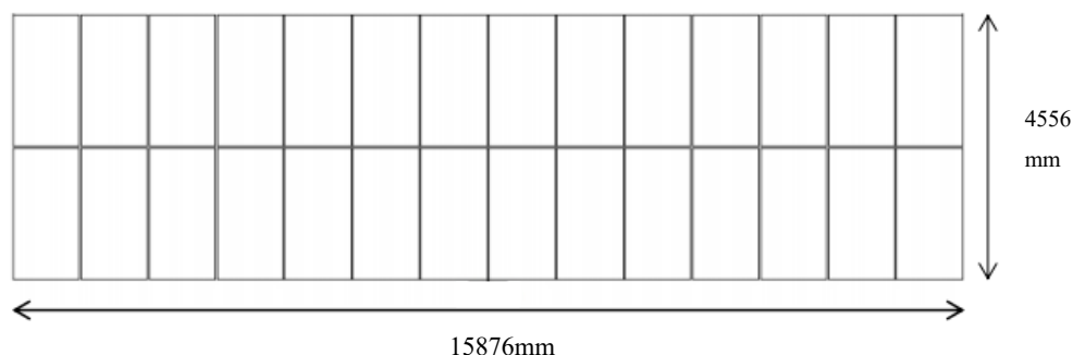
图 2-4 单支架组件排列示意图
