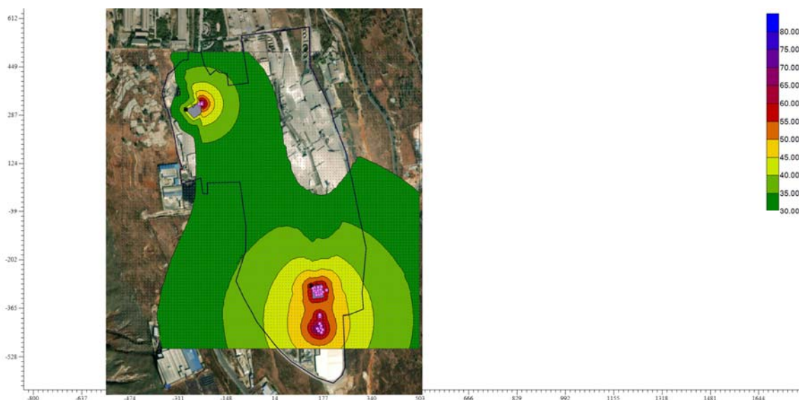
图 4-1 本项目建成运营期噪声贡献等声级线图（昼间及夜间）
