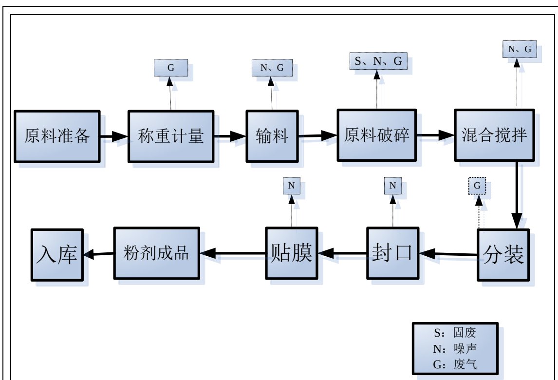
图 4.2 粉剂产品生产工艺流程图
