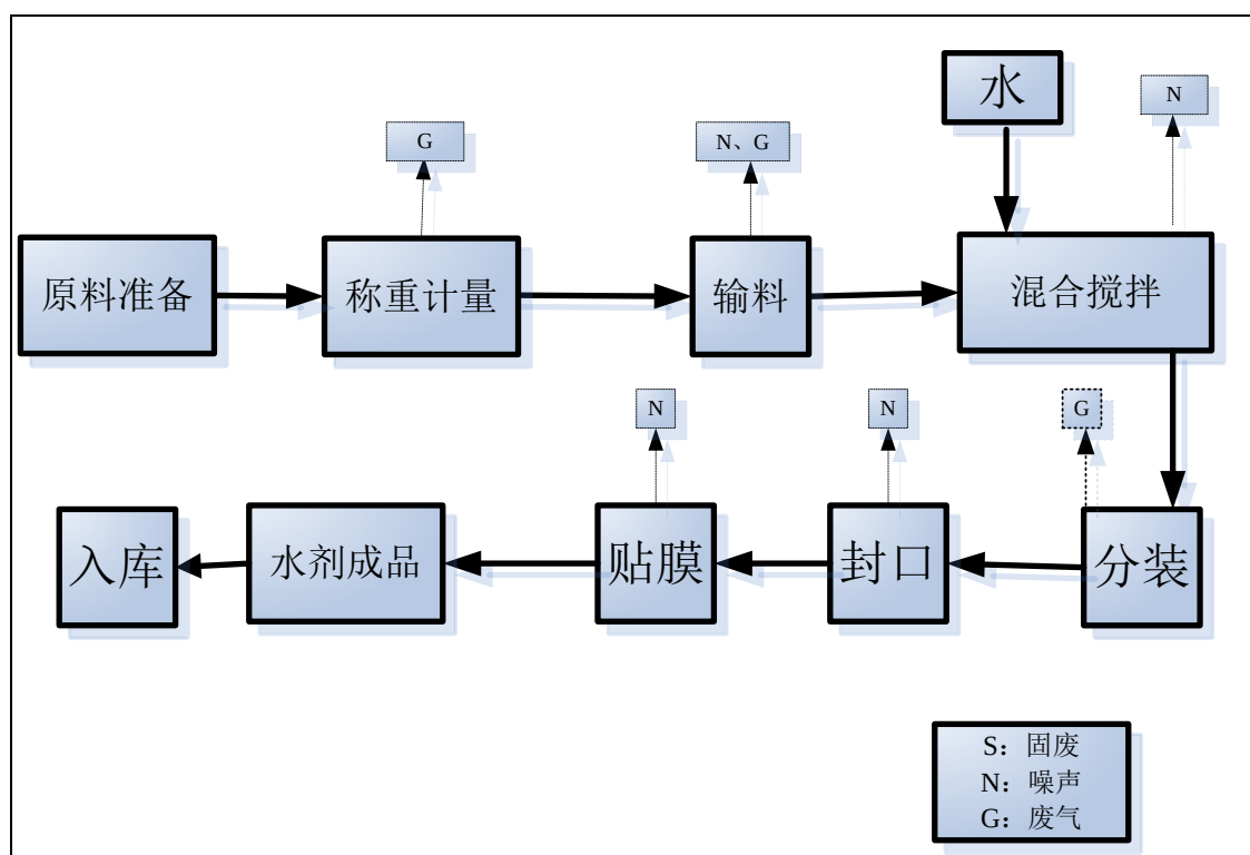
图 4.3 水剂产品生产工艺流程图
