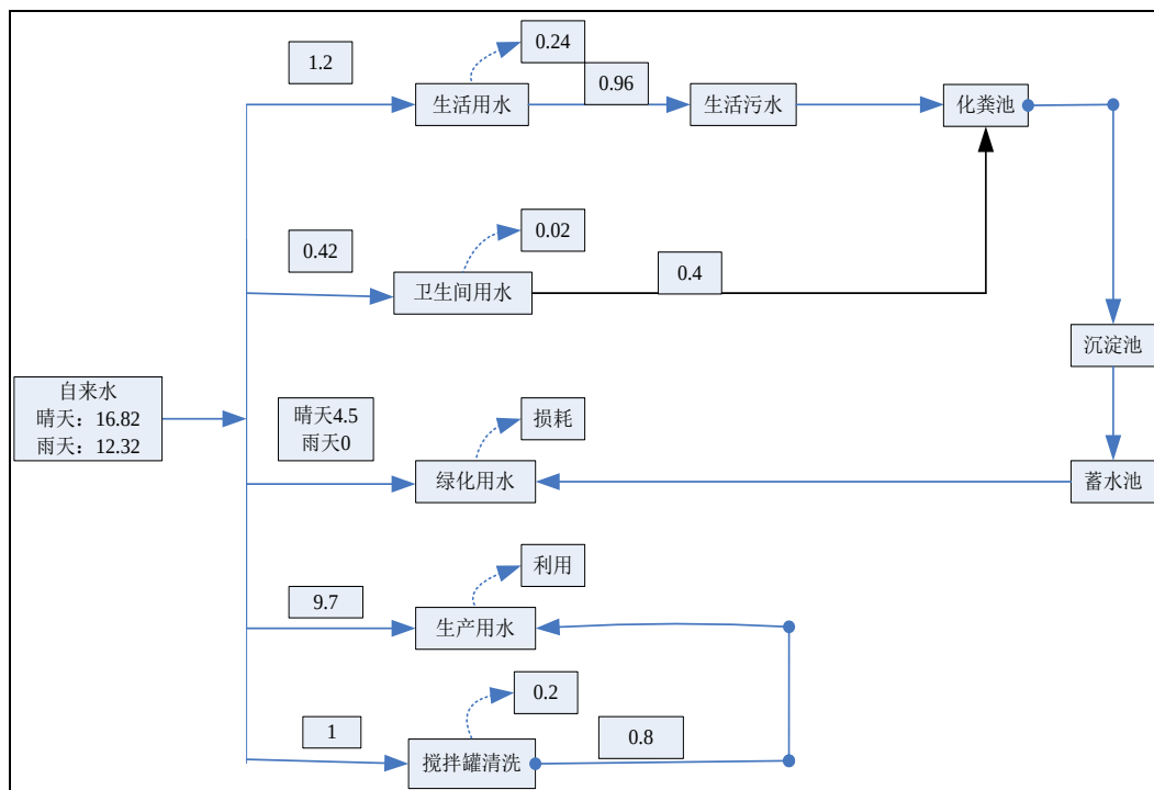
图 4.4 项目近期水平衡图 单位：m³/d
