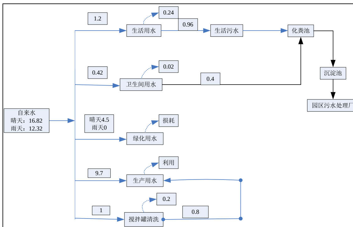
图 4.5 项目远期水平衡图 单位：m³/d
